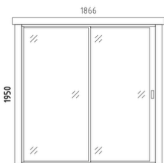
D290-LT | * D290-RT (Aluminium)
